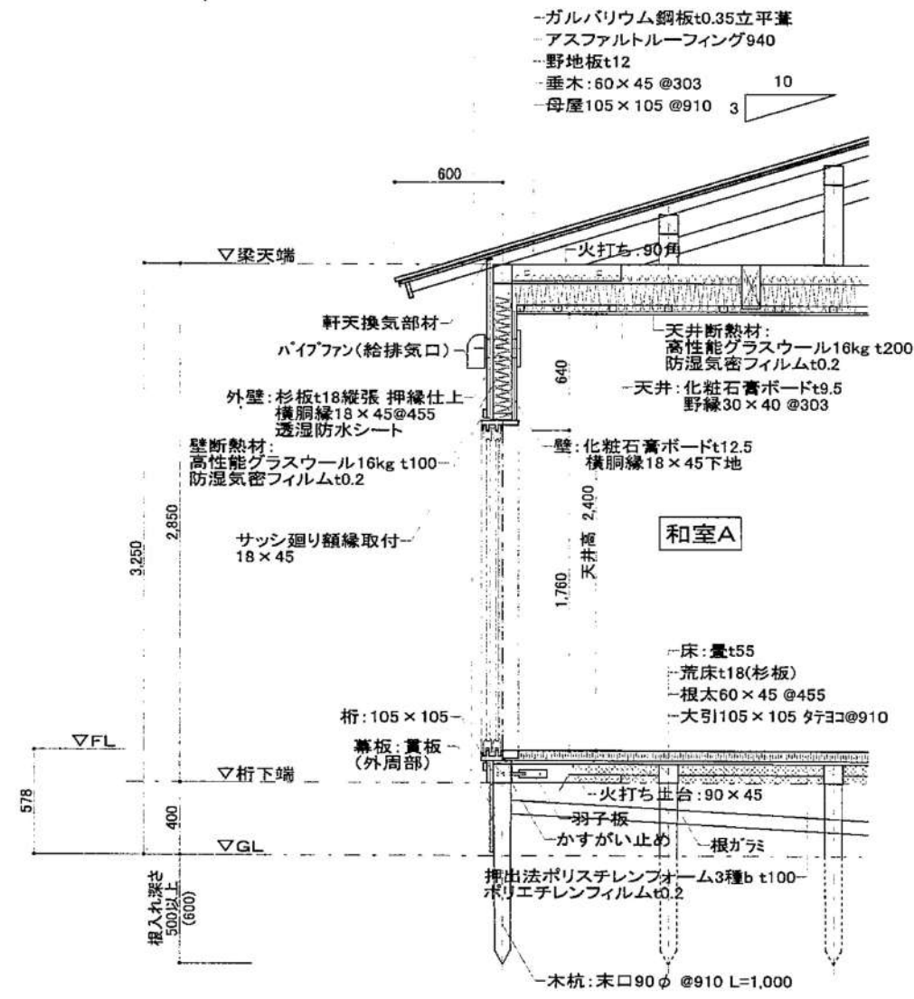
矩計詳細図 S:1/30
