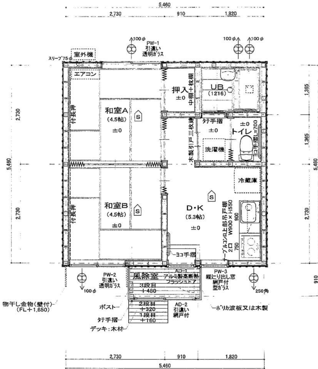
平面詳細図 S:1/50
