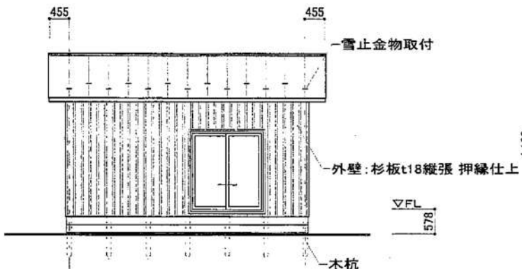
北側立面図 S:1/100
