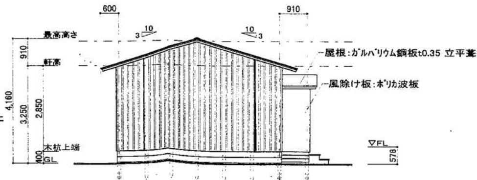
西側立面図 S:1/100
